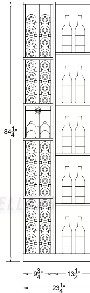
ELEVATION -C-
