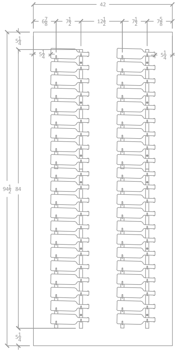
ELEVATION 1 TYP.
